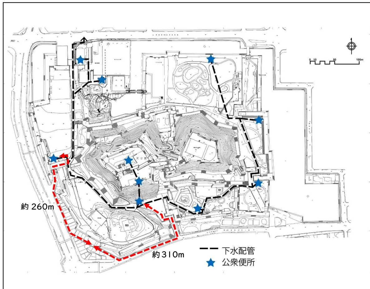
図4-13 既存トイレと扇の芝の位置関係
