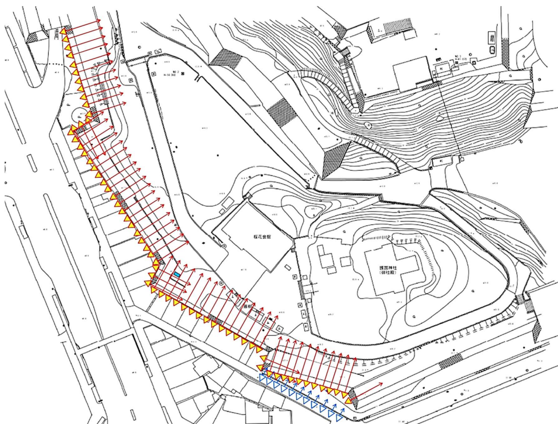
図 4-16 石垣ライトアップ配灯図（案）（パナソニック株式会社エレクトリックワークス社より提供、灯具の種類は次頁参照）
