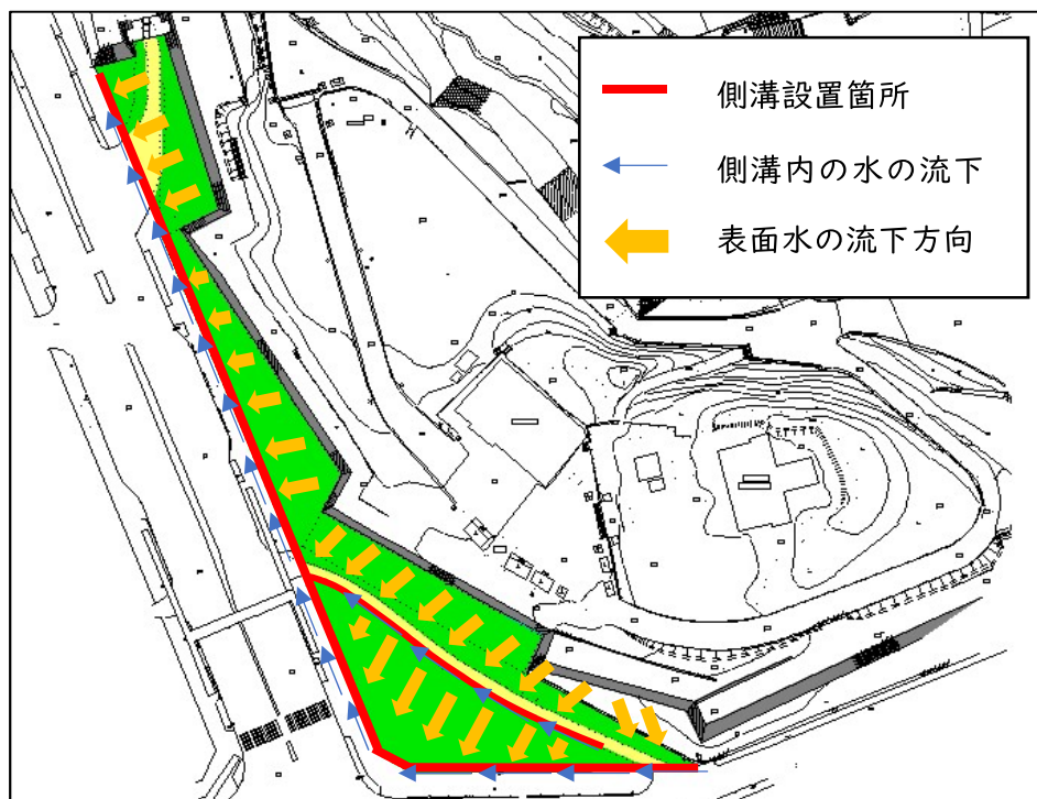
図4-5 排水計画の模式図(例)
