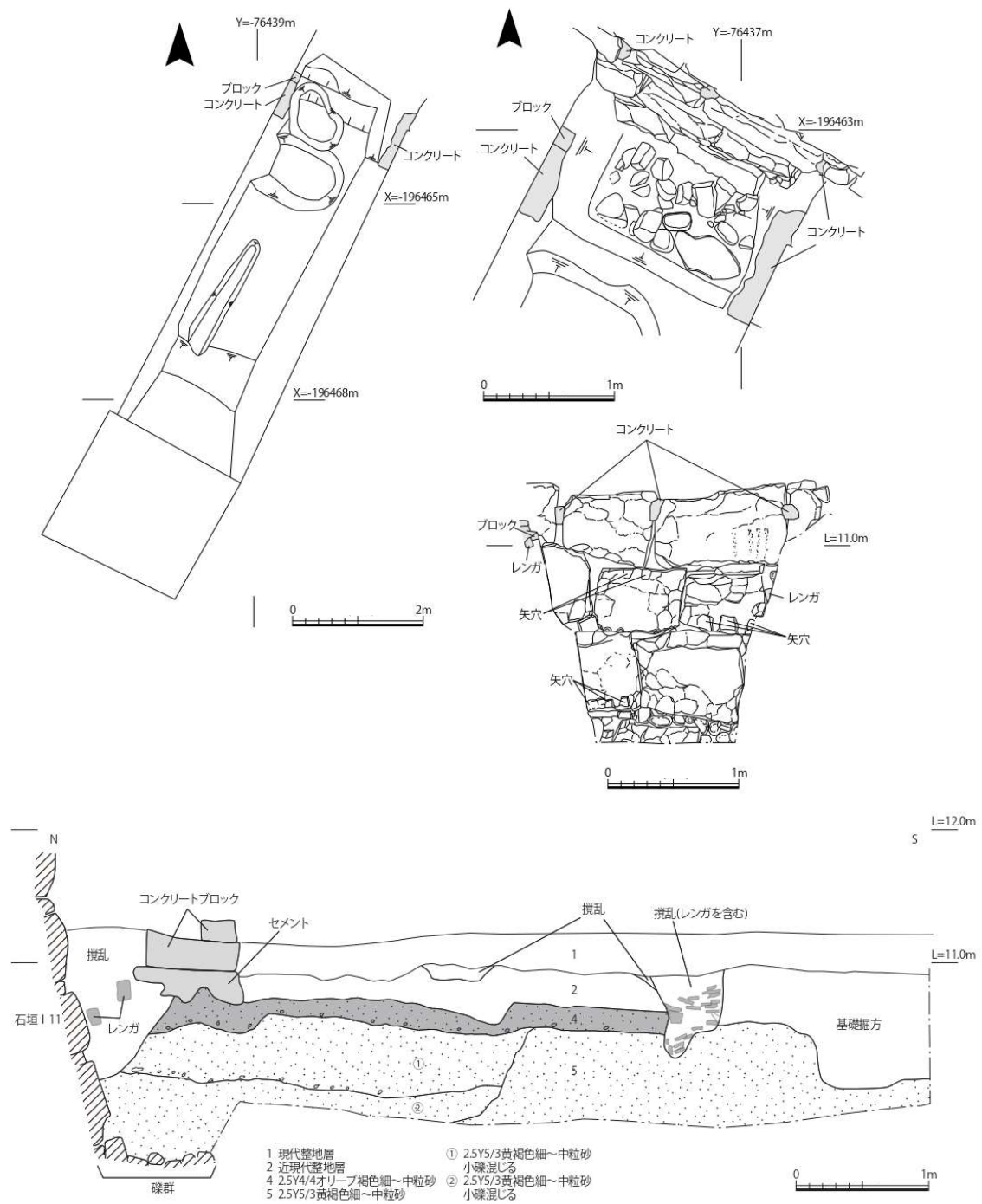
図2-33 2区平面図・石垣ⅡⅠ立面図・南東壁断面図
